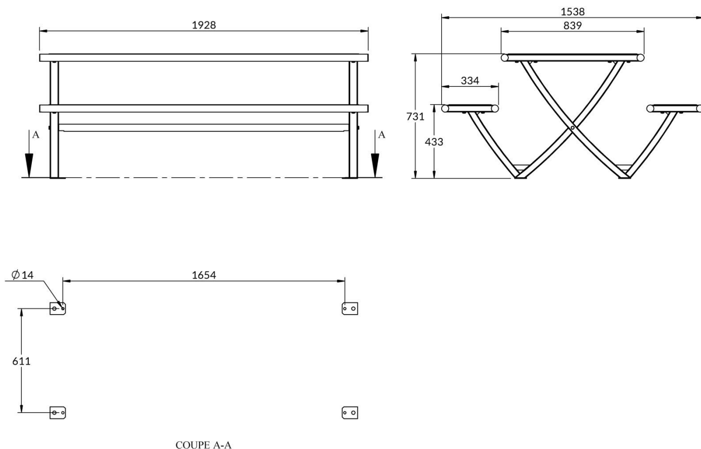
COUPE A-A
